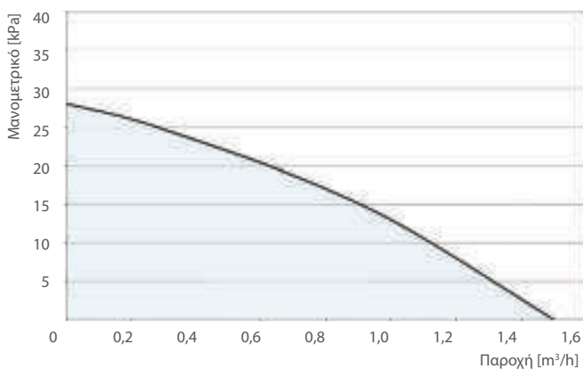
Καμπύλη Απόδοσης D5 Vario 38/700 B
