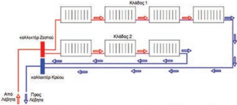
Ενδεικτικό σχέδιο μονοσωληνίου συστήματος θέρμανσης
