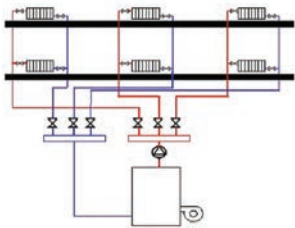
Ενδεικτικό σχέδιο δισωληνίου συστήματος θέρμανσης
