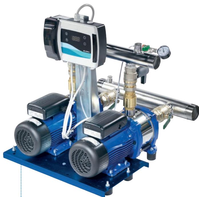
Σειρά GXS: Μονοφασικά με μεταδότες πίεσης
